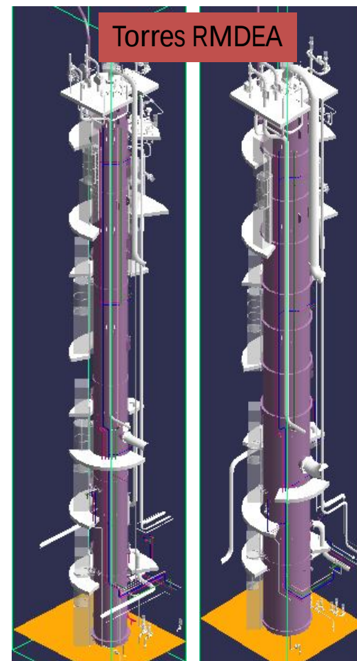
Seção U-38
